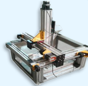
اسکنر تست آلتراسونیک HIC
