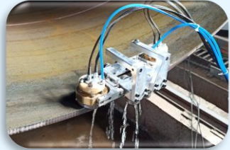
اسکنر تست التراسونیک انتهای لوله
